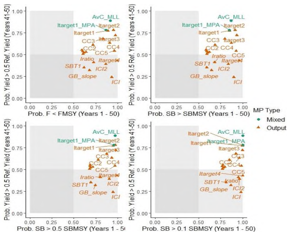
Рисунок 14 – Оценка эффективности стратегий управления при определении величины ОДУ стерляди в водных объектах Томской области с использованием программы DLMtool
