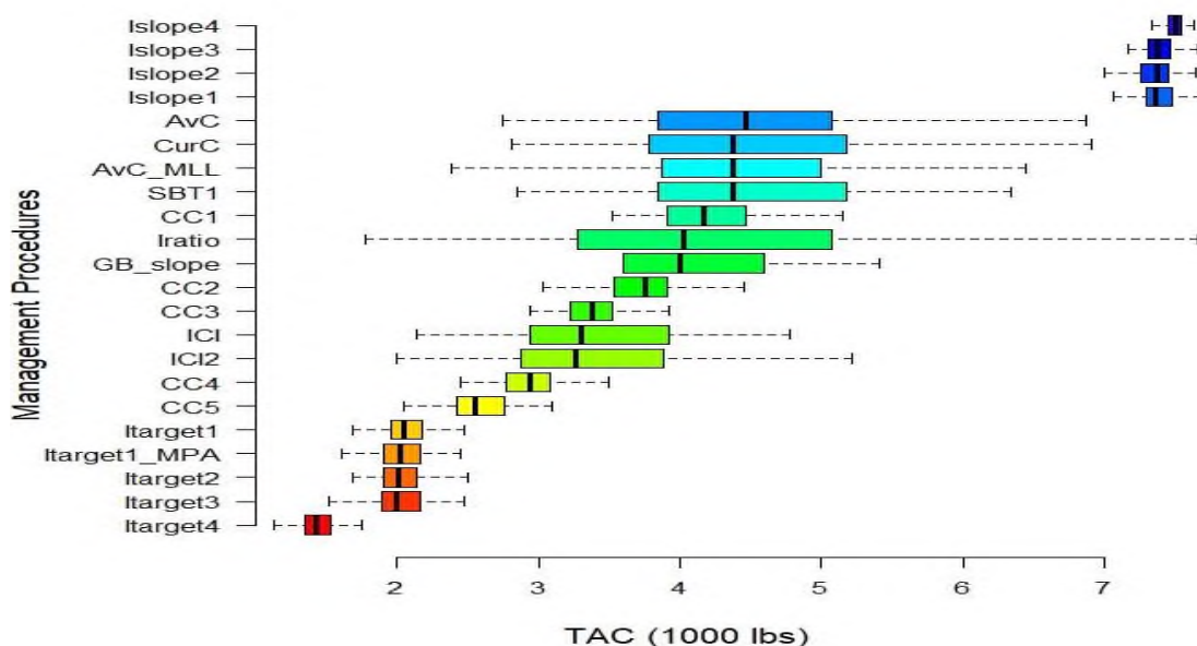
Рисунок 13 – Диапазон оценок ОДУ применяемых процедур управления к запасам стерляди в водных объектах Томской области с использованием программы DLMtool
