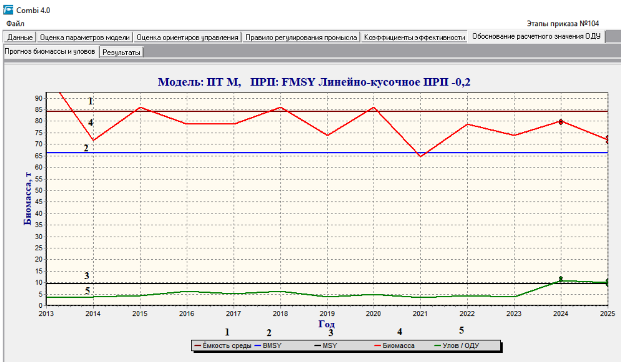
Рисунок 9 – Прогноз биомассы и ОДУ стерляди в водных объектах Томской области на 2024-2025 гг. с использованием программы COMBI 4.0
