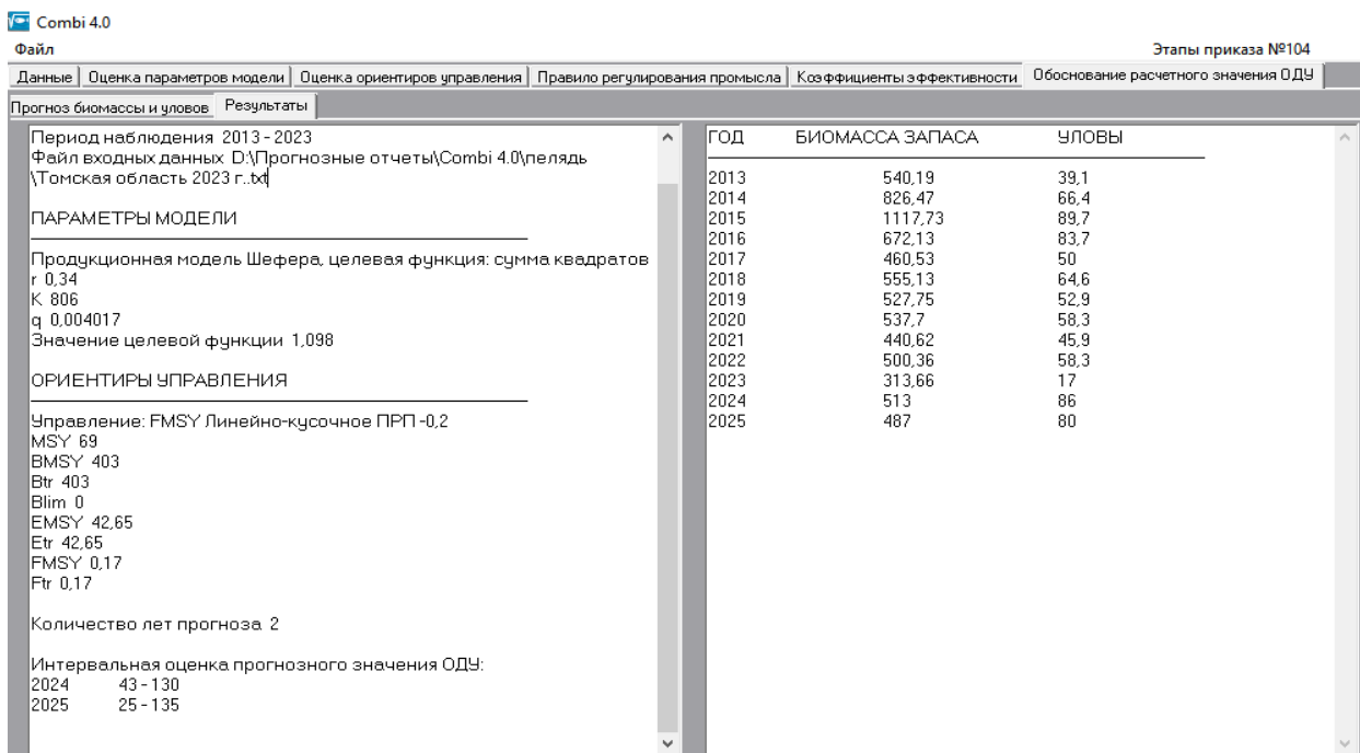
Рисунок 31 – Результаты обоснования расчетного значения ОДУ пеляди в водных объектах с использованием программы СОМБИ 4.0
