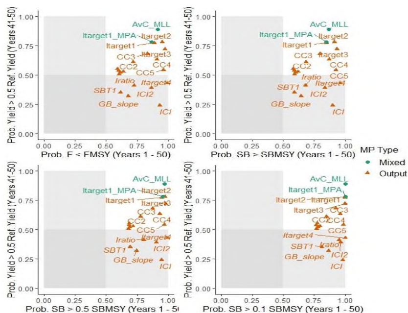
Рисунок 24 – Оценка эффективности стратегий управления при определении величины ОДУ нельмы в водных объектах Томской области с использованием программы DLMtool
