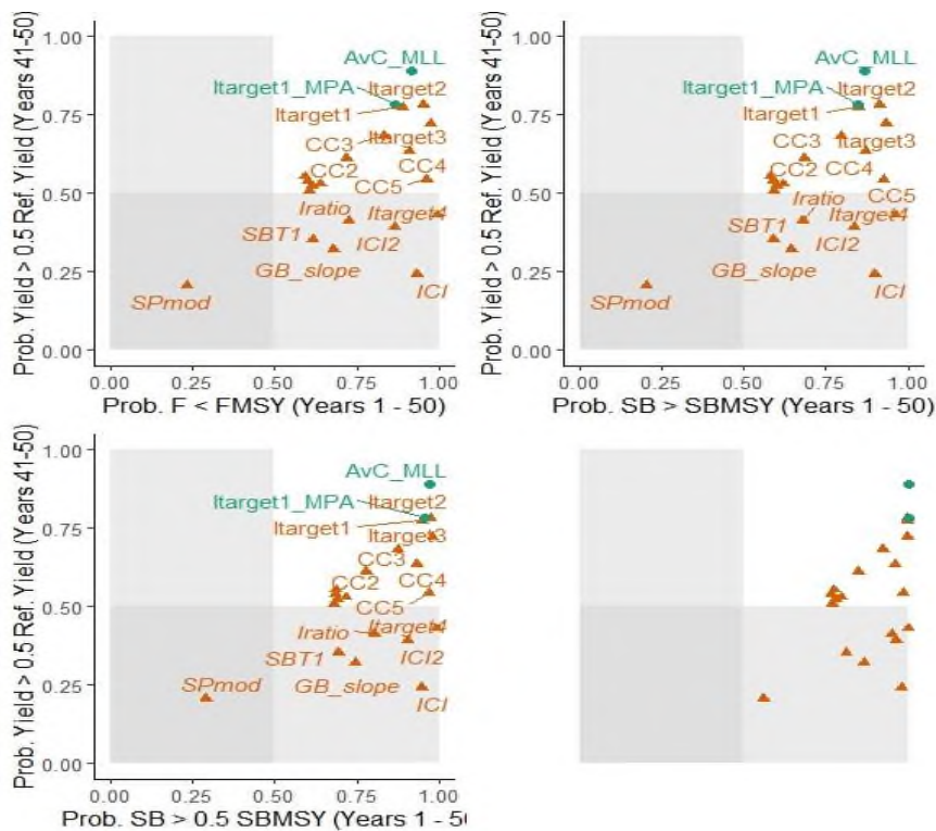
Рисунок 33 – Оценка эффективности стратегий управления при определении величины ОДУ пеляди в водных объектах Томской области с использованием программы DLMtool
