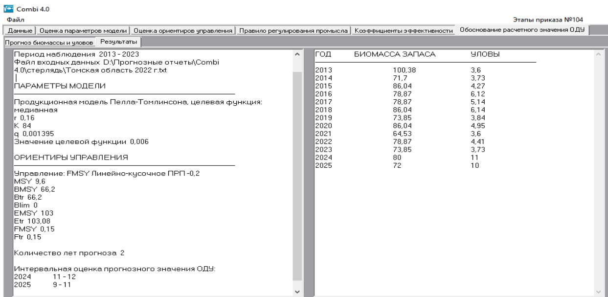
Рисунок 12 – Результаты обоснования расчетного значения ОДУ стерляди в водных объектах Томской области с использованием программы COMBI 4.0
