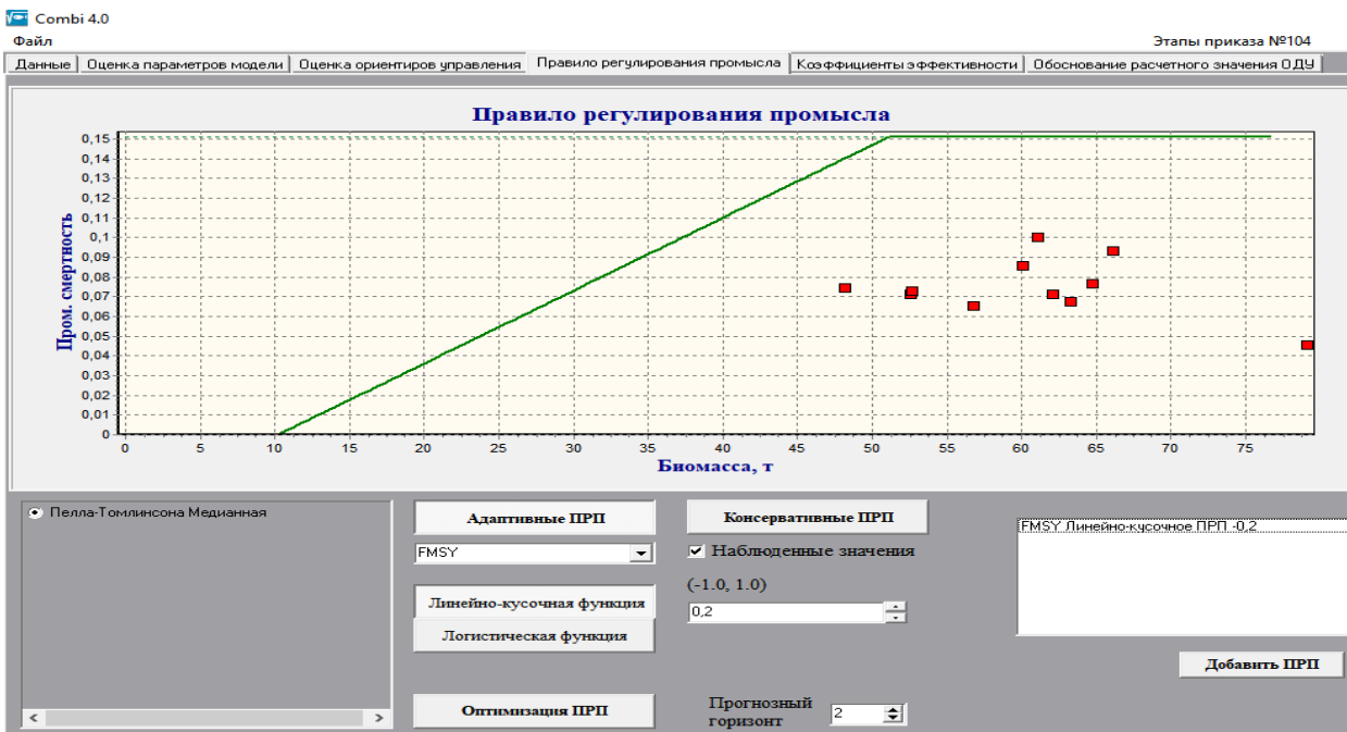
Рисунок 10 – Правило регулирования промысла стерляди в водных объектах Томской области на 2025 г. с использованием программы COMBI 4.0
