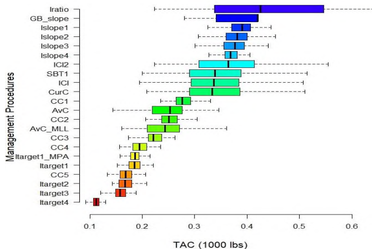
Рисунок 18 – Диапазон оценок ОДУ применяемых процедур управления к запасам муксуна в водных объектах Томской области с использованием программы DLMtool
