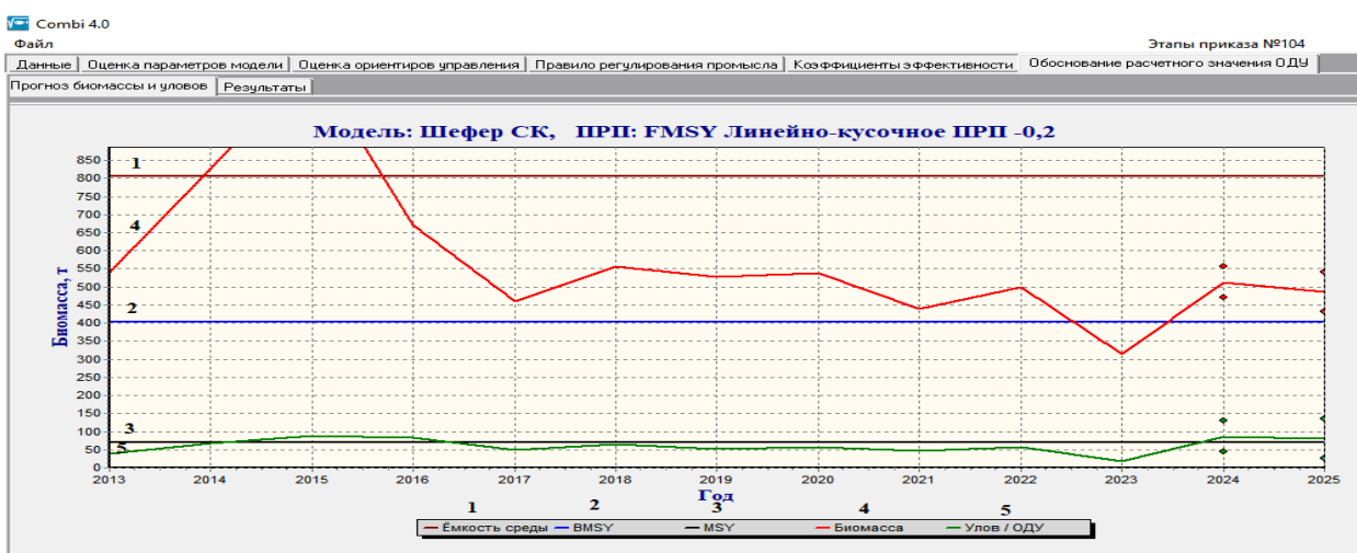
Рисунок 28 – Прогноз биомассы и ОДУ пеляди в водных объектах Томской области на 2024-2025 гг. с использованием программы COMBI 4.0
