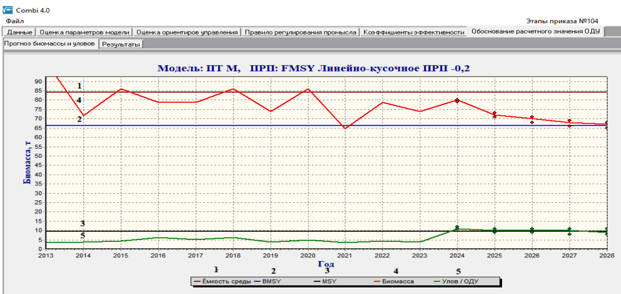
Рисунок 11 – Прогноз состояния биомассы и ОДУ стерляди в водных объектах Томской области на 2025-2028 гг. с использованием программы COMBI 4.0
