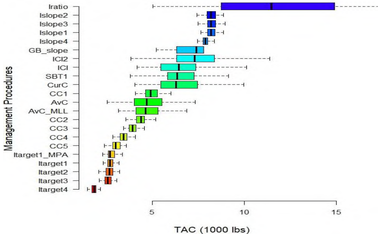
Рисунок 13 – Диапазон оценок ОДУ применяемых процедур управления к запасам стерляди в водных объектах Томской области с использованием программы DLMtool
