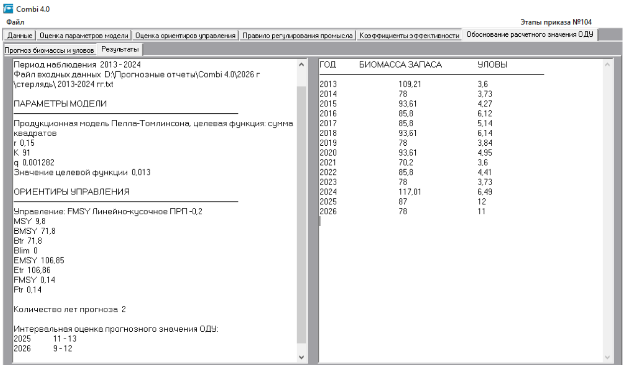
Рисунок 12 – Результаты обоснования расчетного значения ОДУ стерляди в водных объектах Томской области с использованием программы COMBI 4.0
