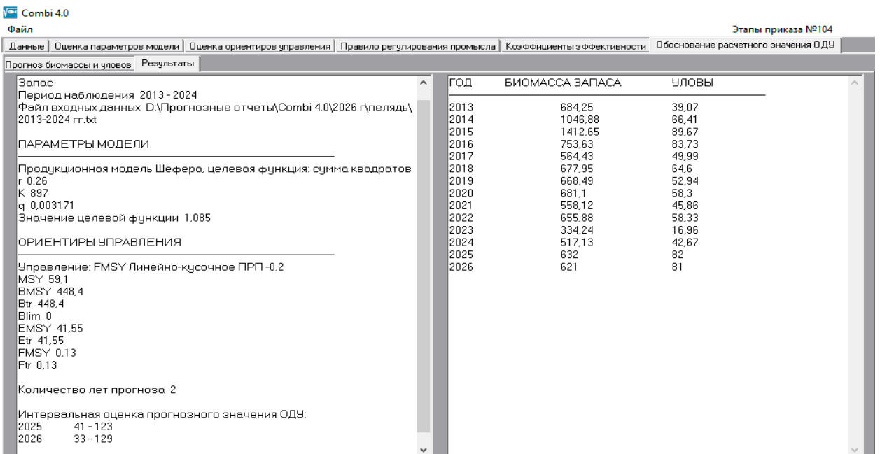
Рисунок 31 – Результаты обоснования расчетного значения ОДУ пеляди в водных объектах с использованием программы СОМБИ 4.0
