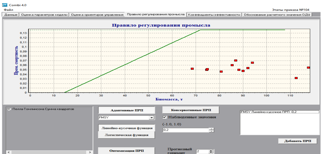
Рисунок 10 – Правило регулирования промысла стерляди в водных объектах Томской области на 2026 г. с использованием программы COMBI 4.0
