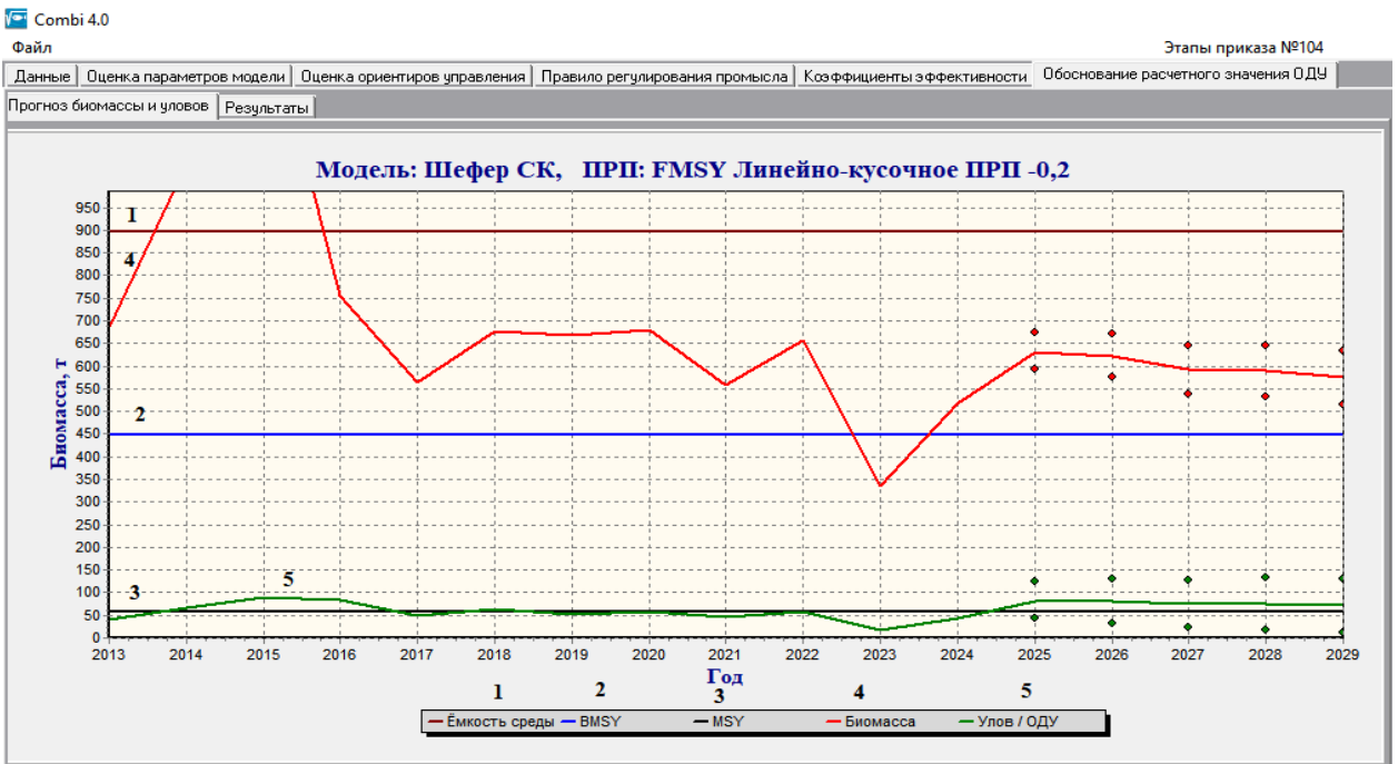
Рисунок 30 – Прогноз состояния биомассы и ОДУ пеляди на 2026–2029 гг. с использованием программы СОМБИ 4.0
