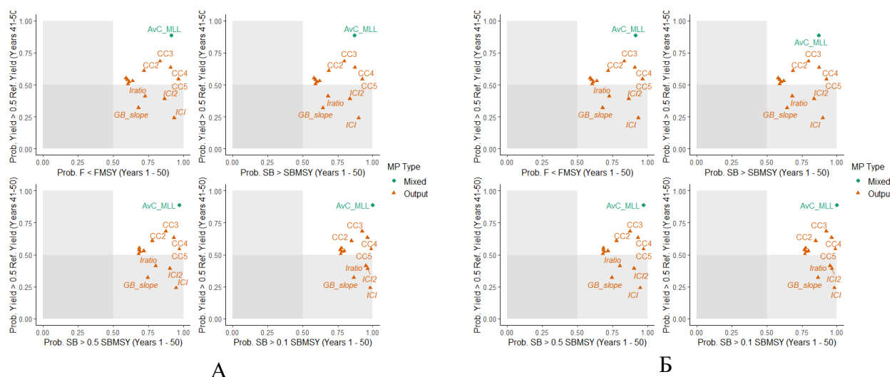
Рисунок 6 – Оценка эффективности стратегий управления при определении величины ОДУ стерляди с использованием программы DLMtool р. Оби в Сузунском районе (А) и в нижнем бьефе НГЭС (Б)
