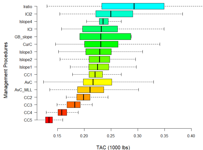
Рисунок 7 – Диапазон оценок ОДУ применяемых процедур управления с использованием программы DLMtool к запасу нельмы р. Оби в нижнем бьефе НГЭС
